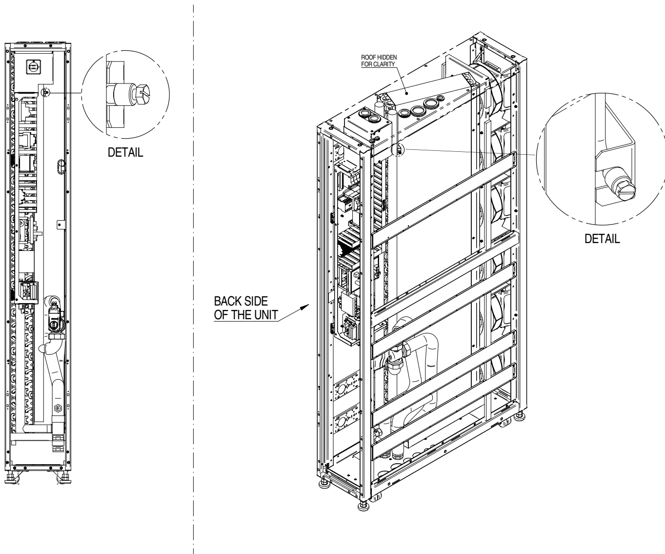
Fig. 8e Air bleeding valve position CW
