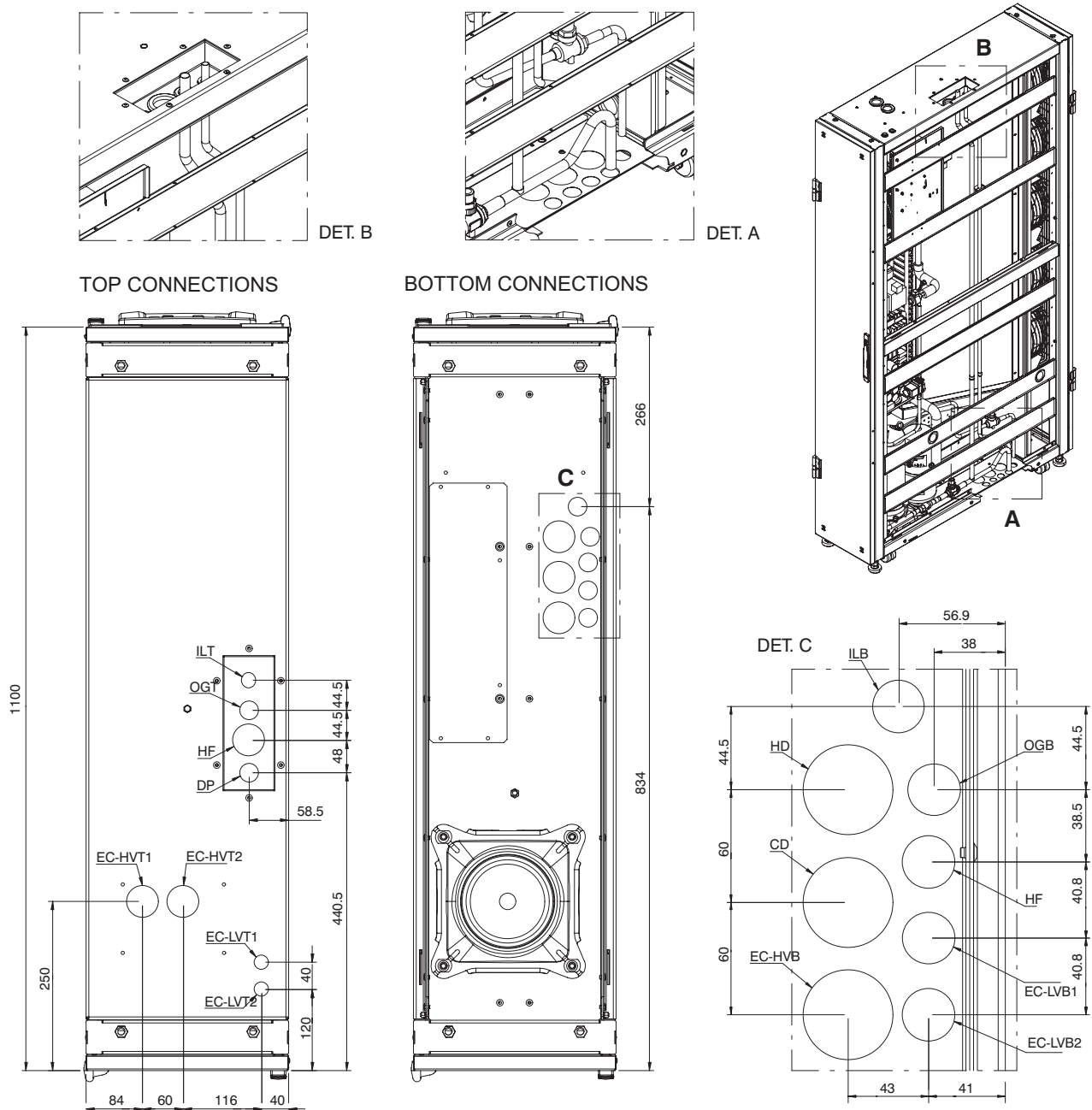
Fig. 9a CR011RA - CR021RA connections
