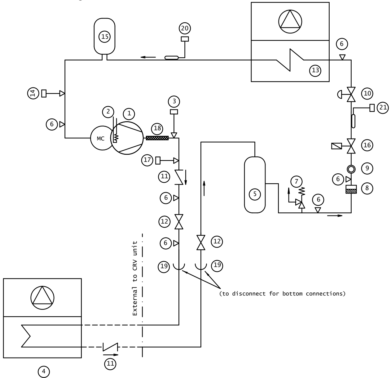
Fig. 10a Liebert CR011RA - CR021RA
